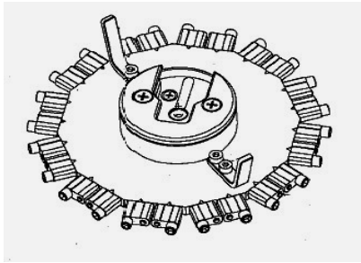
Φ1.25フェルル24本V溝研磨治具
