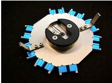
LCフェルル研磨治具
