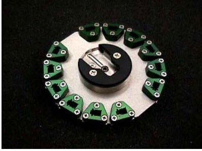
LCプラグ斜め研磨治具(8°)
