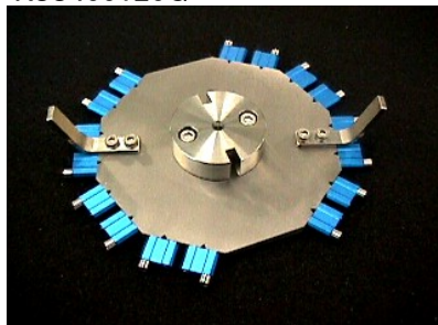
LCエルール研磨治具
