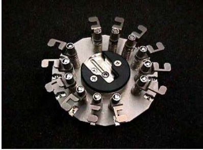
MUプラグAPC研磨治具
