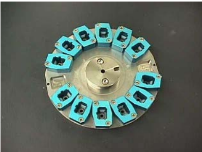
SCプラグ研磨治具
