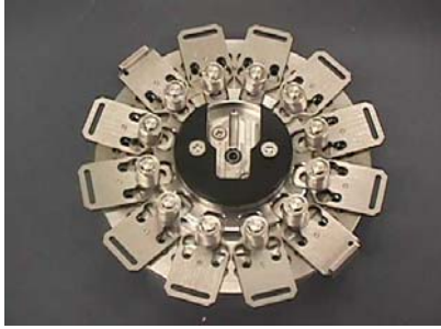
24本取り斜め8度用研磨治具(縦突起)
