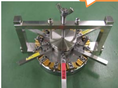
MT再研磨用高さ合わせ治具 * MT研磨治具は含まれておりません。 HCB250
