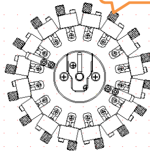
φ2.5フェルール用8度斜め研磨治具(16本)
