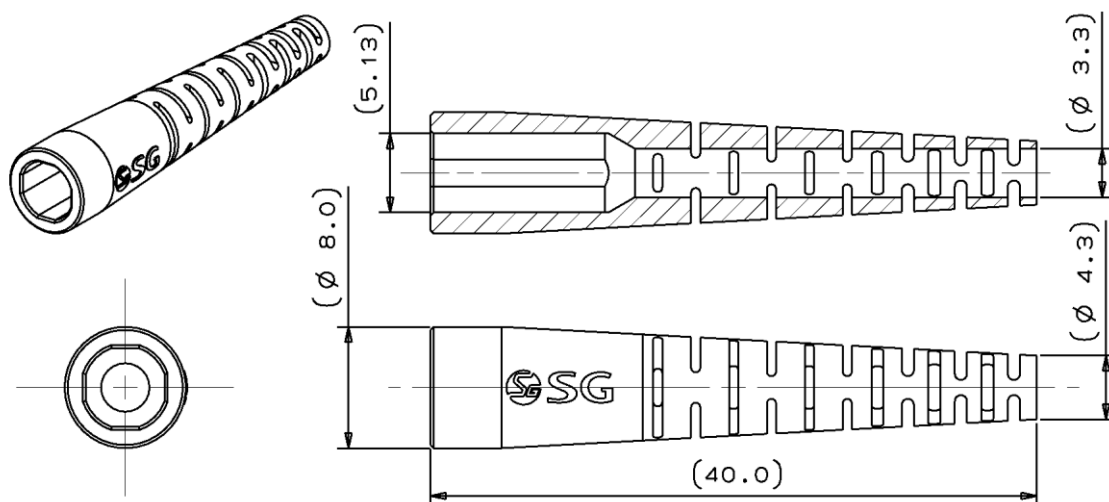
図 14. ⑦-1 ブーツ (φ3 mm コード用)
