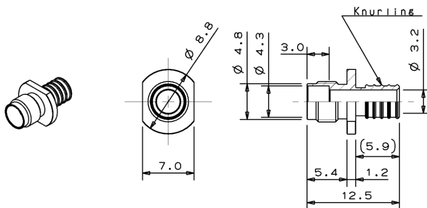
図 9. ④ストッパ
