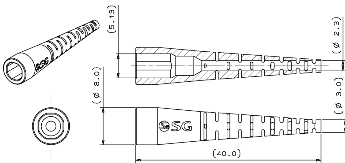
図 15. ⑦-2 ブーツ (φ2 mm コード用)
