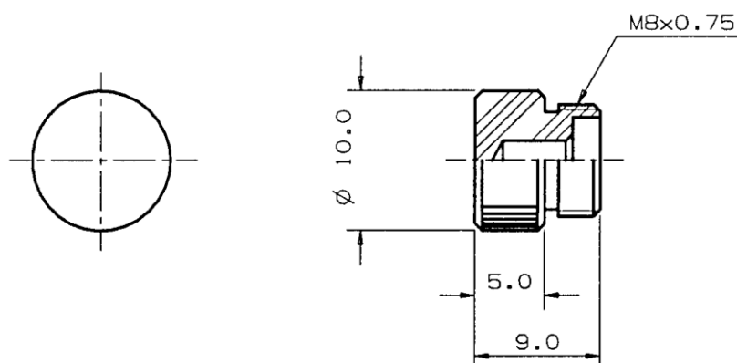
図 18. ⑧-3 キャップ (プラスチックキャップ)
