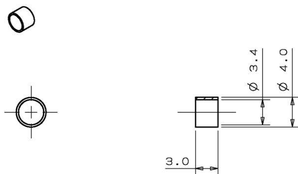
図 13. ⑥-2 リング (ø 2 mm コード用)
