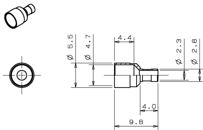
図 11. ⑤-2 カシメリング (ø 2 mm コード用)
