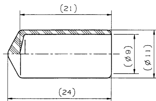
図 17. ⑧-2 キャップ (帽子キャップ)
