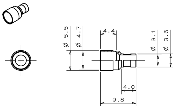
図 10. ⑤-1 カシメリング (ø 3 mm コード用)
