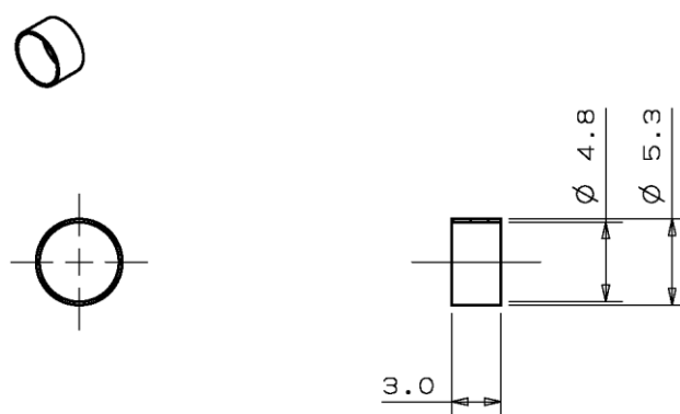
図 12. ⑥-1 リング (ø 3 mm コード用)
