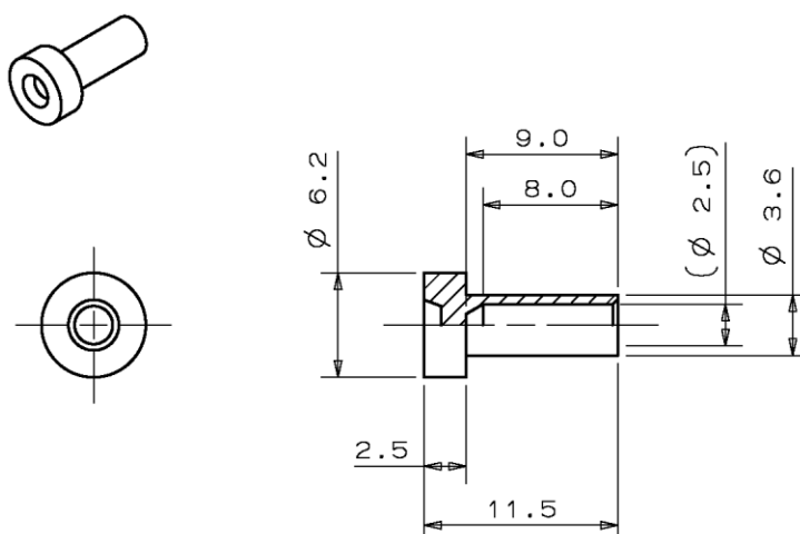
図 16. ⑧-1 キャップ (フェルールキャップ)
