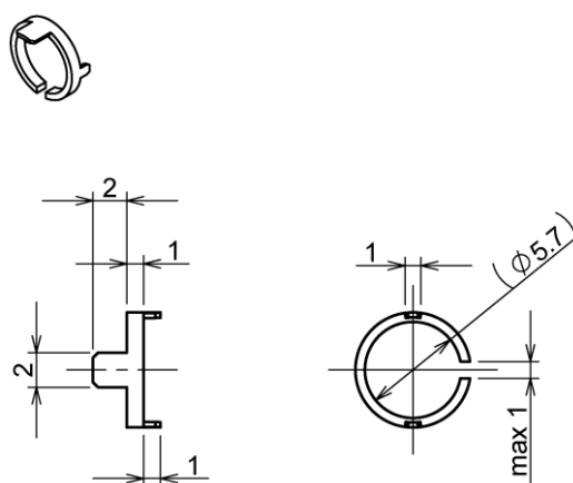
図3 ②キーリング
