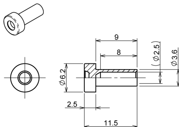
図7 ⑥キャップ (フェルールキャップ)
