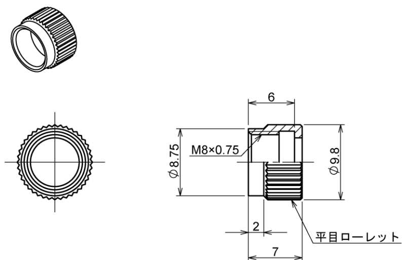
図5 ④カップリングナット
