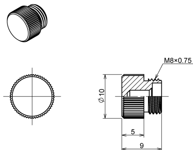
図8 ⑧キャップ (プラスチックキャップ)
