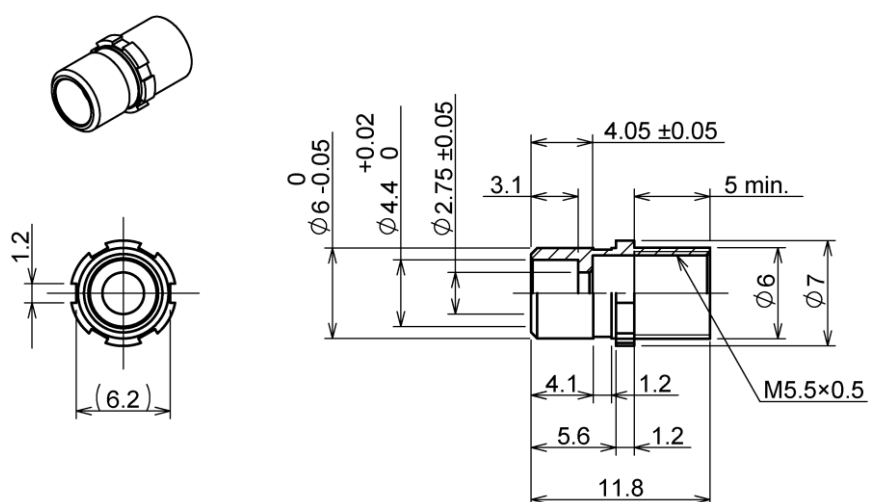
図 2 ①フレーム
