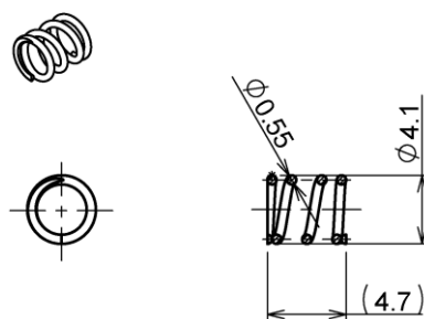
図 4 ③スプリング
