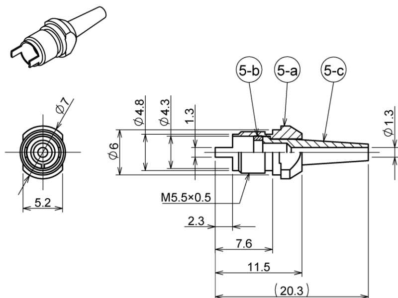
図6 ⑤ストッパ
