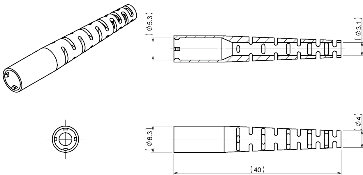
図 11 ⑦-1 ブーツ(φ 3 mm コード用)
