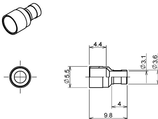
図7 ⑤-1 カシメリング(φ3 mm コード用)
