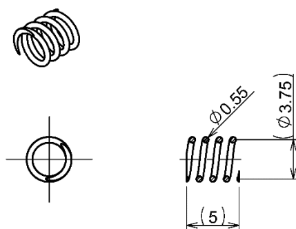
図 5 ③スプリング
