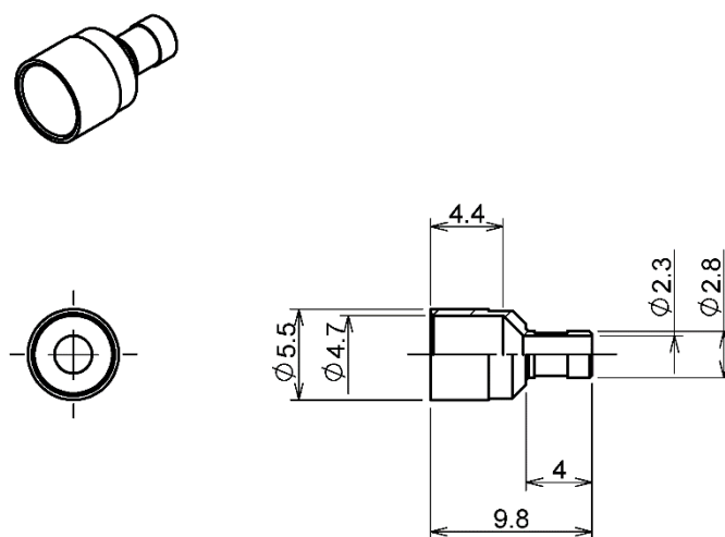
図8 ⑤-2 カシメリング(φ2 mm コード用)
