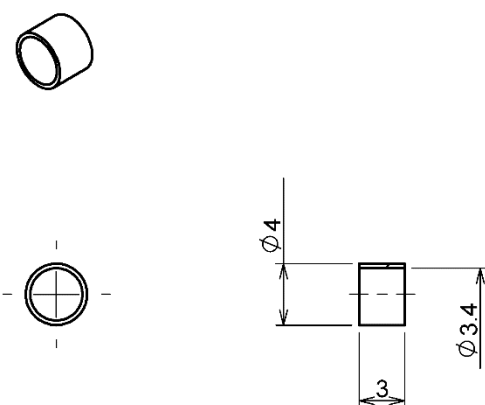
図 9 ⑥-1 リング(φ 3 mm コード用)
