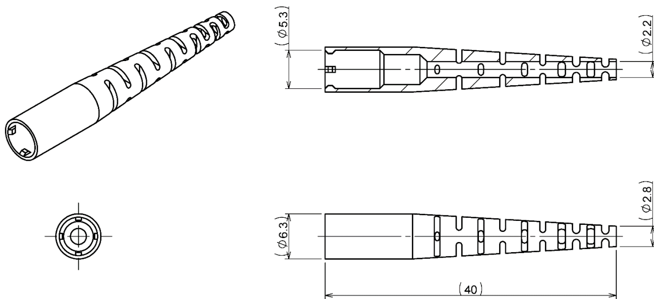
図 11 ⑦-1 ブーツ(φ 3 mm コード用)
