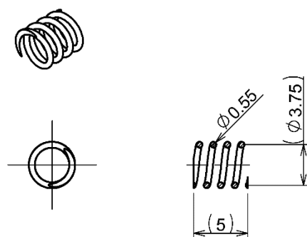
図 5 ③スプリング
