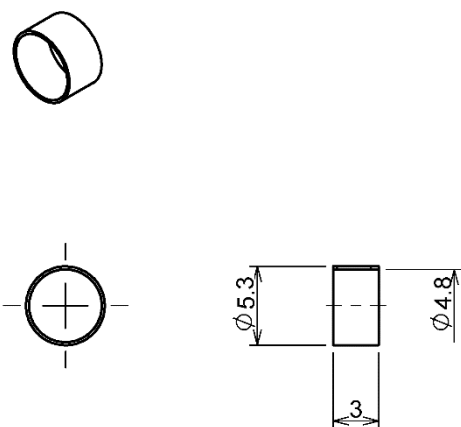
図 9 ⑥-1 リング(φ 3 mm コード用)
