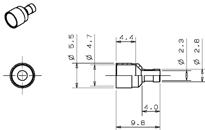
図 6 ⑤カシメリング
