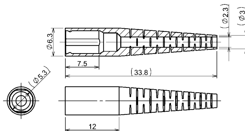
図 8 ⑦ブーツ (ショートタイプ)
