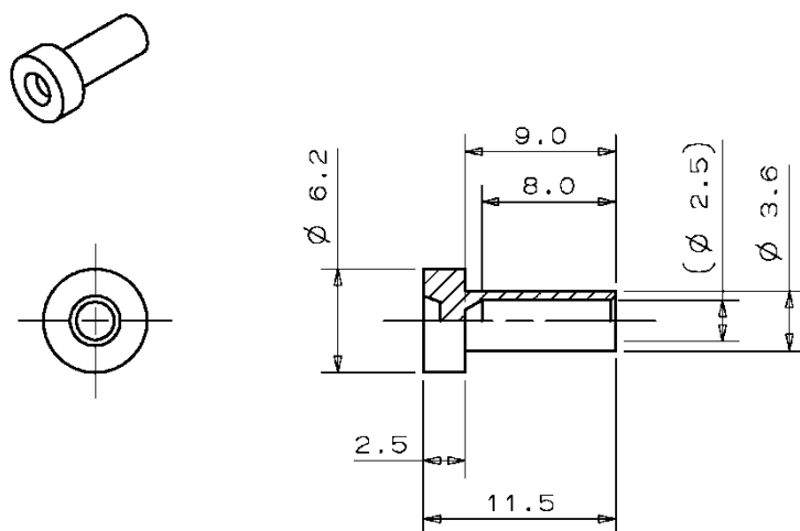
図 9 ⑧-1 キャップ (フェルールキャップ)
