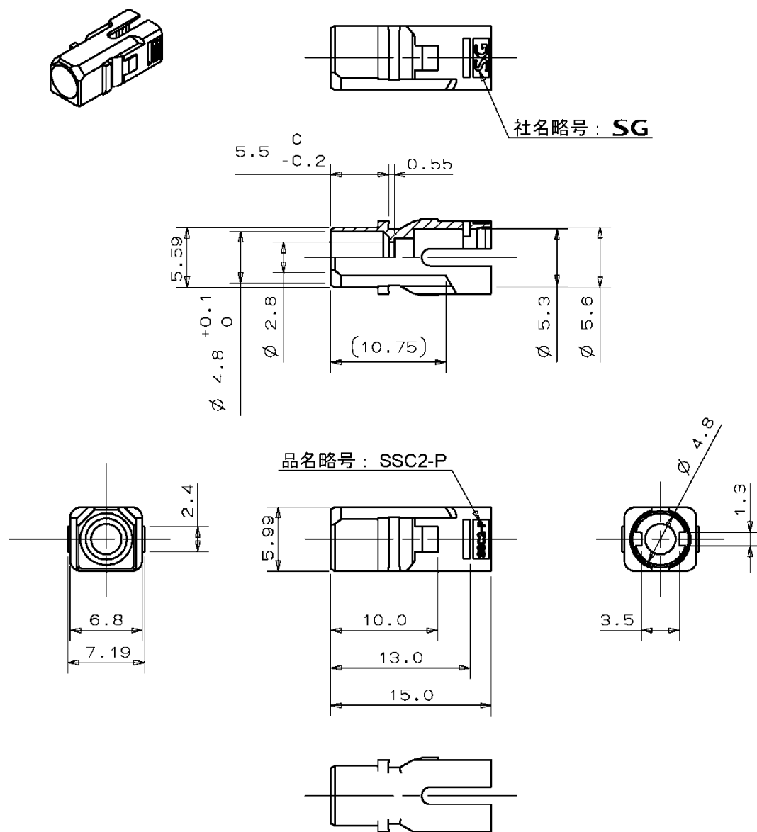
図3 ②プラグフレーム
